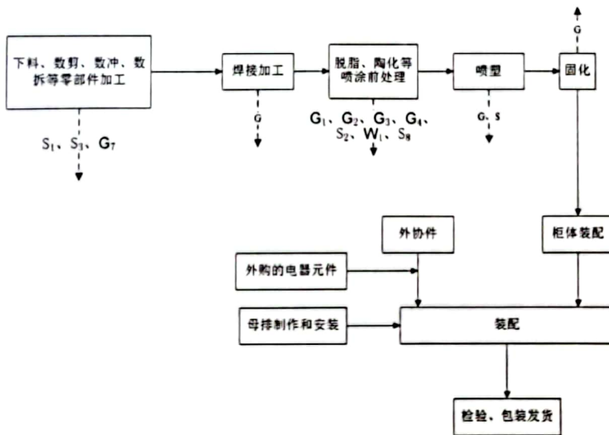
图 3-2 主要生产工艺流程示意图
